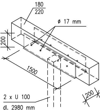
měřítko 1:25
